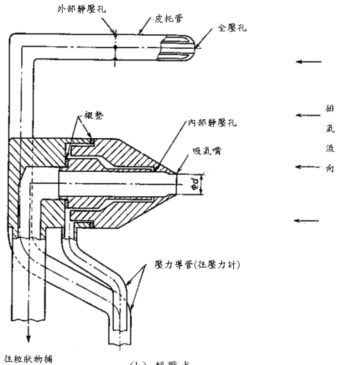
(b) 靜壓式
