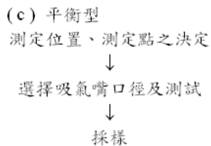
圖十四 粒狀物採樣流程
