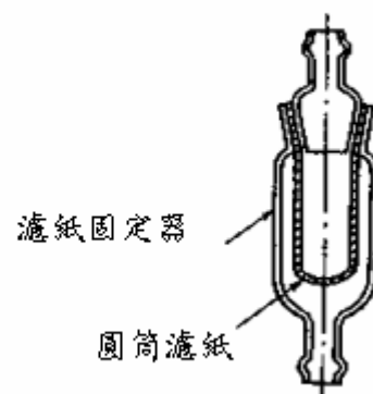
(b) 2 型
