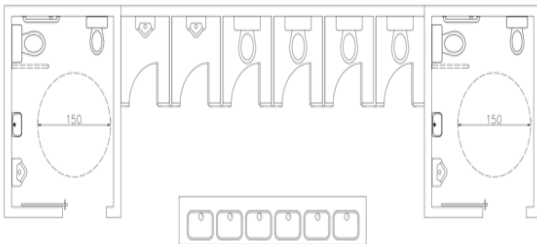
圖 2. 型態 2(圖片來源：內政部性別友善廁所設計指引第 6 頁)
