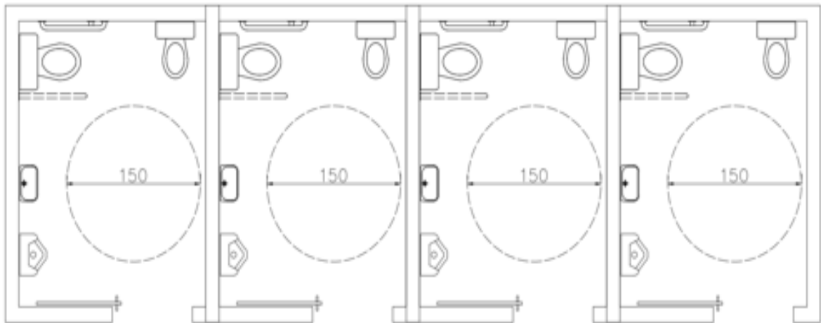
圖 3. 型態 3(圖片來源：內政部性別友善廁所設計指引第 6 頁)
