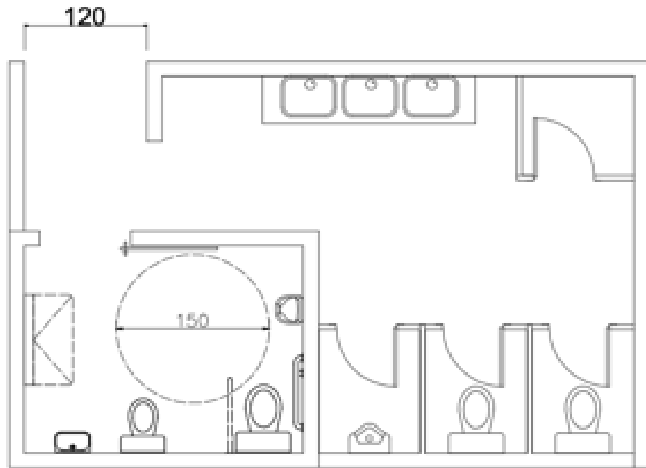
圖 1. 型態 1(圖片來源：內政部性別友善廁所設計指引第 7 頁)
