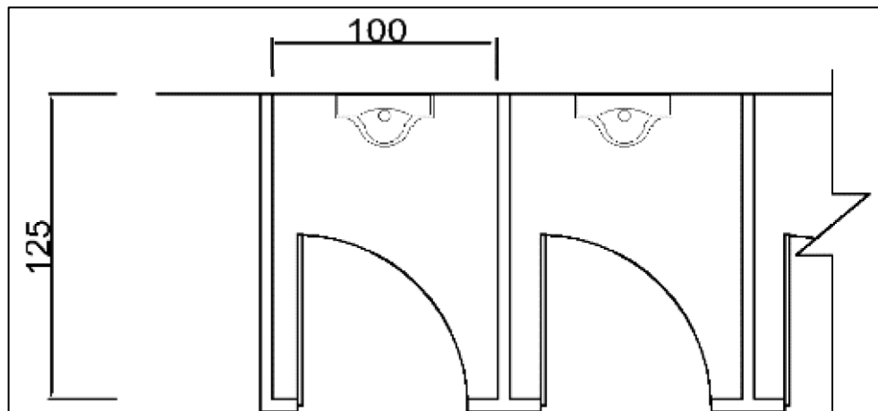
圖 4、小便器廁間空間尺寸
