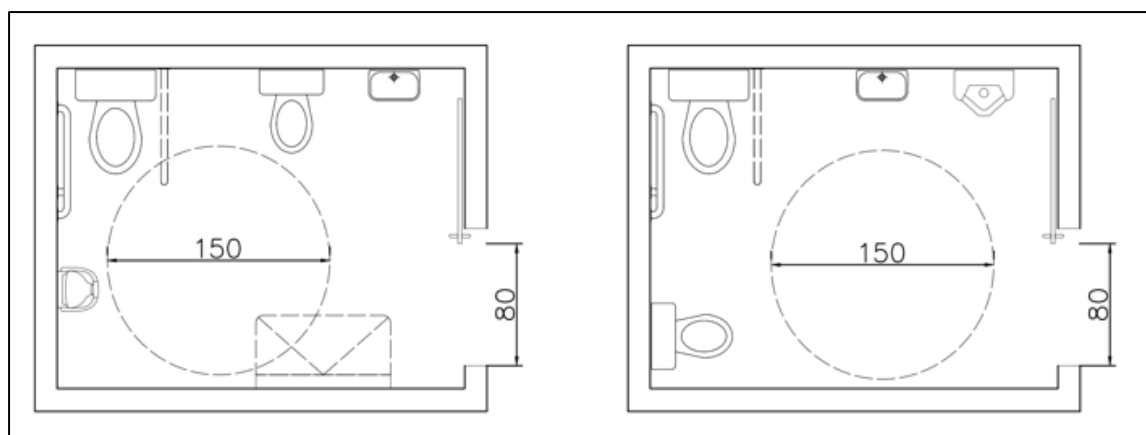
圖 5、獨立式多功能廁所空間尺寸
