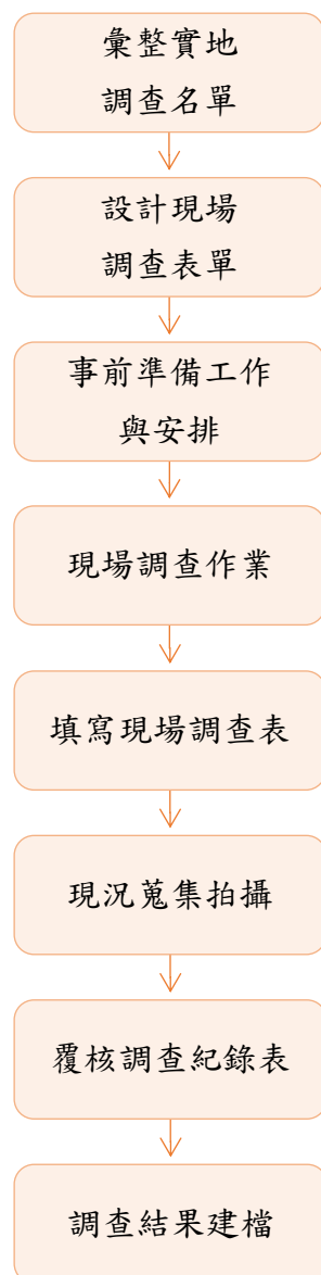
圖 2.2-1 含石綿建材建築物現況調查作業流程圖
