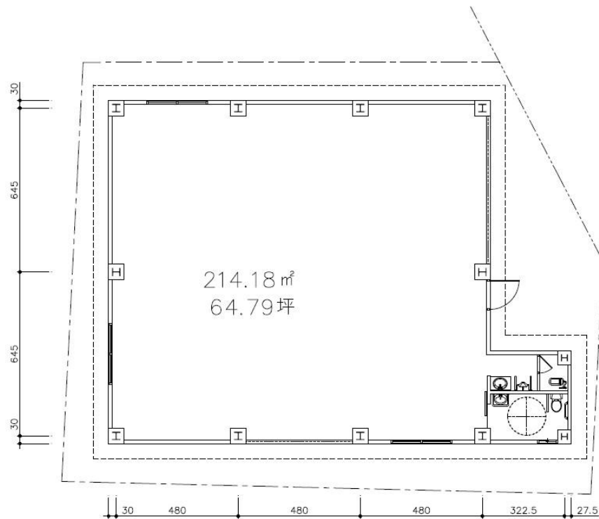
圖 3.1-8 暫存場之平面配置圖
