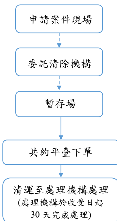
圖 2.3-2 石綿建材廢棄物清除處理流程
