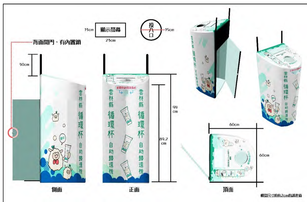
圖 3.5-2 自助歸還機機體設計
